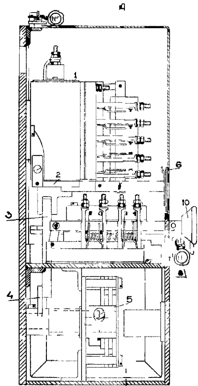
DOORSNEDE C-D
