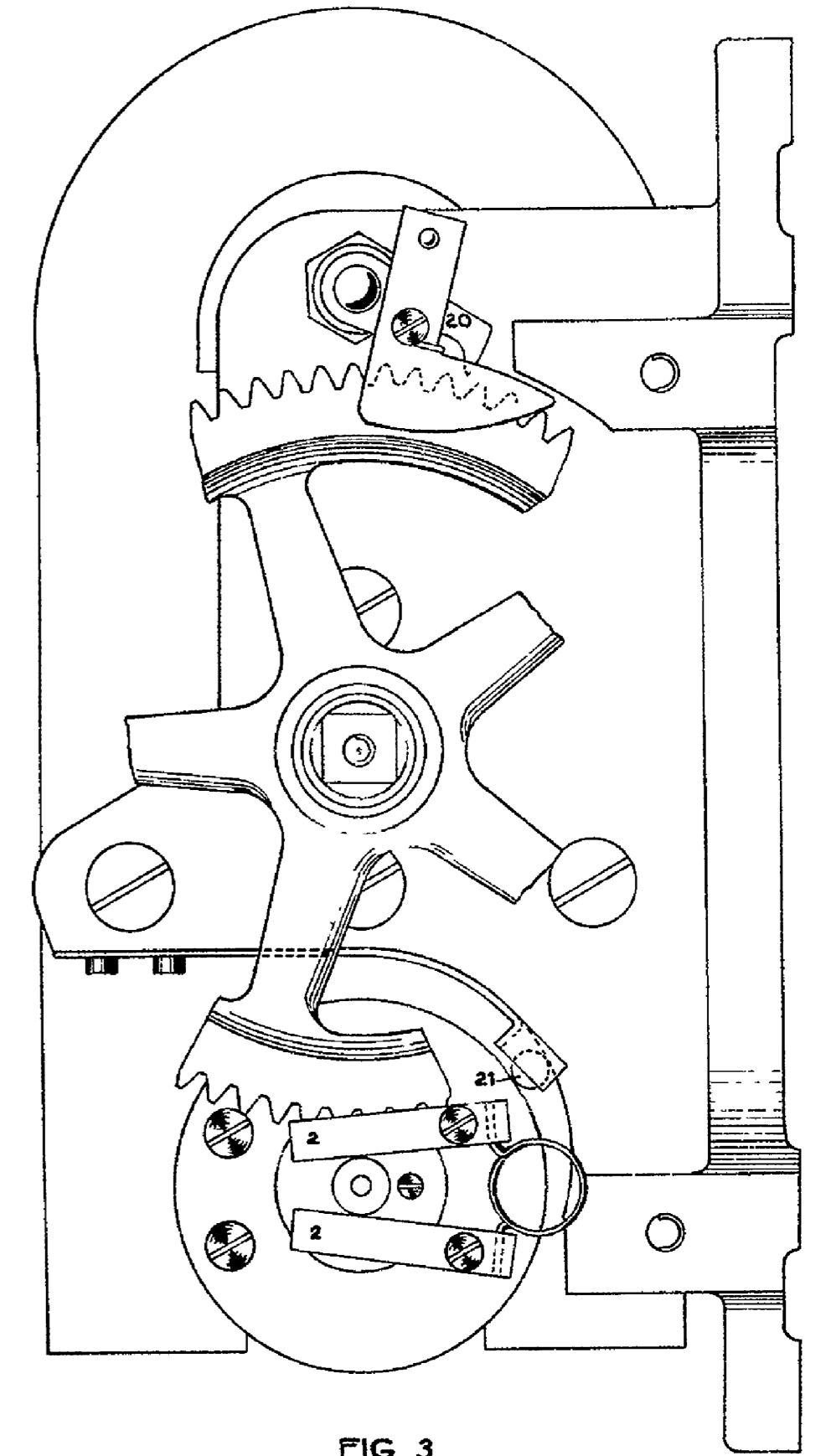
FIG. 3 SLUITSTUK VAN FRAME AFGENOMEN.
