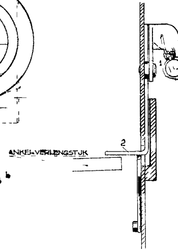
DOORSNEDE A-B
